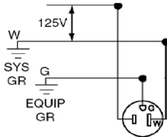
Diagrama de cableado
