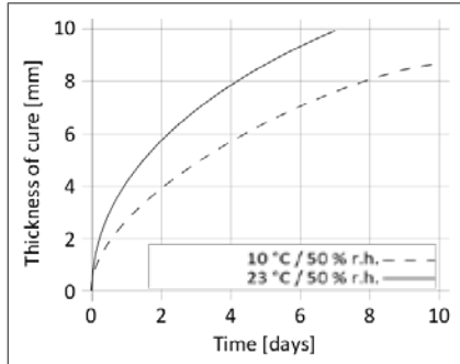
Diagrama 1: Velocidad de curado Sikaflex® SOLO
