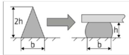
Figura 1: Configuración recomendada del cordón
